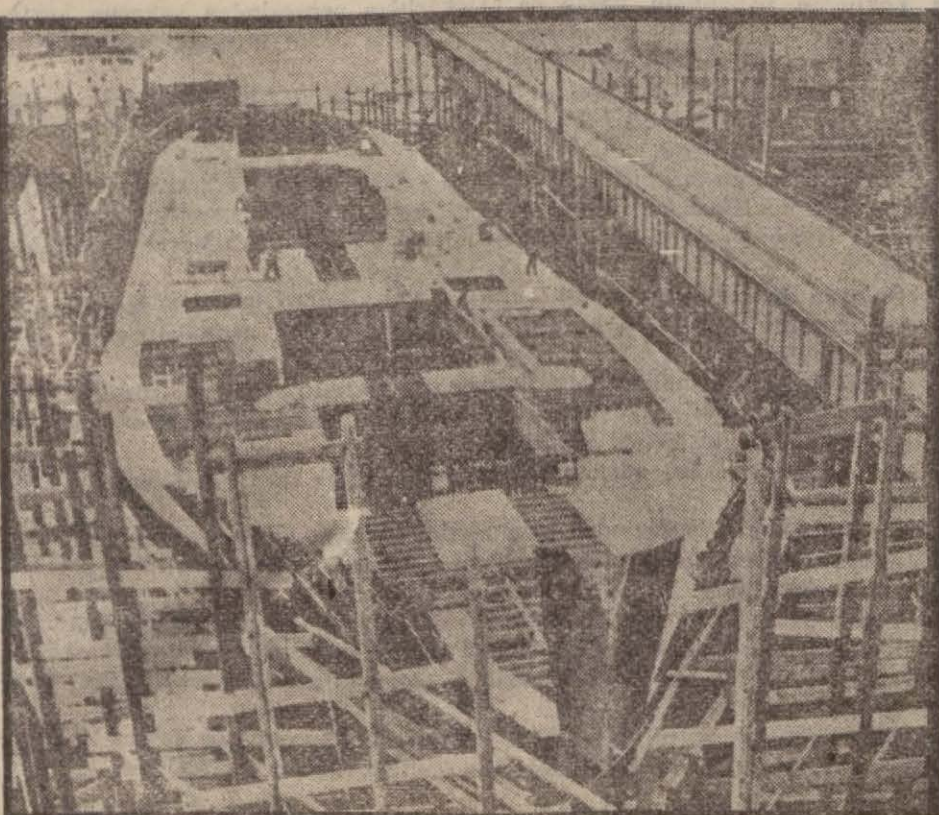
Kanada tersanelerinde yapılmakta olan bir geminin çelik kaburgası
